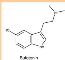
Bufotenin
